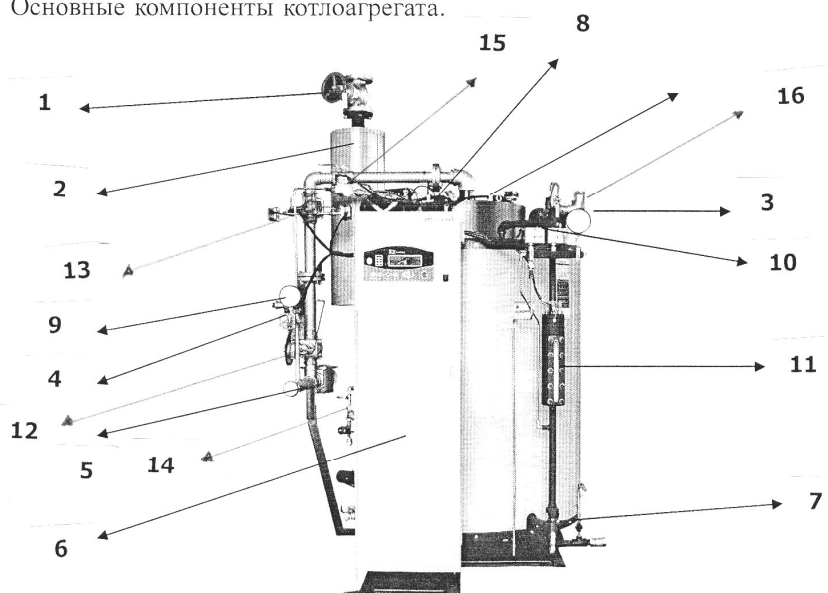
Основные компоненты котлоагрегата.
